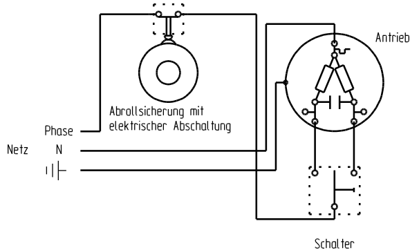
Beispiel 1 : Anschluß an einen Schalter
