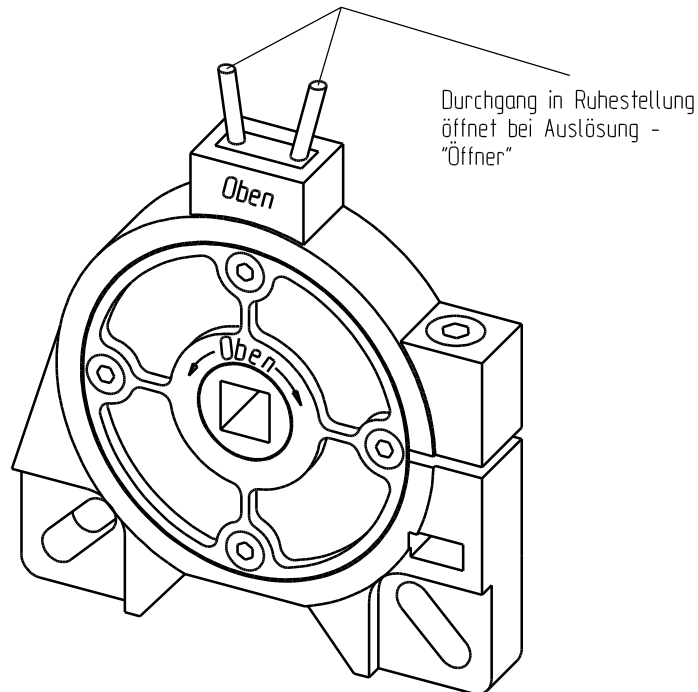
Beispiel 2 : Anschluß an eine Steuerung
